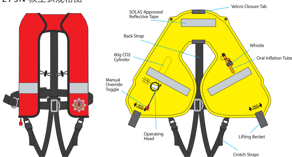
275N 救生衣规格图
